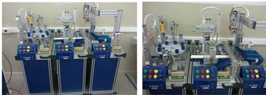
Fig. AIV-4 - Conjunto Mecatrônico integrado a Supervisão de Processo.
